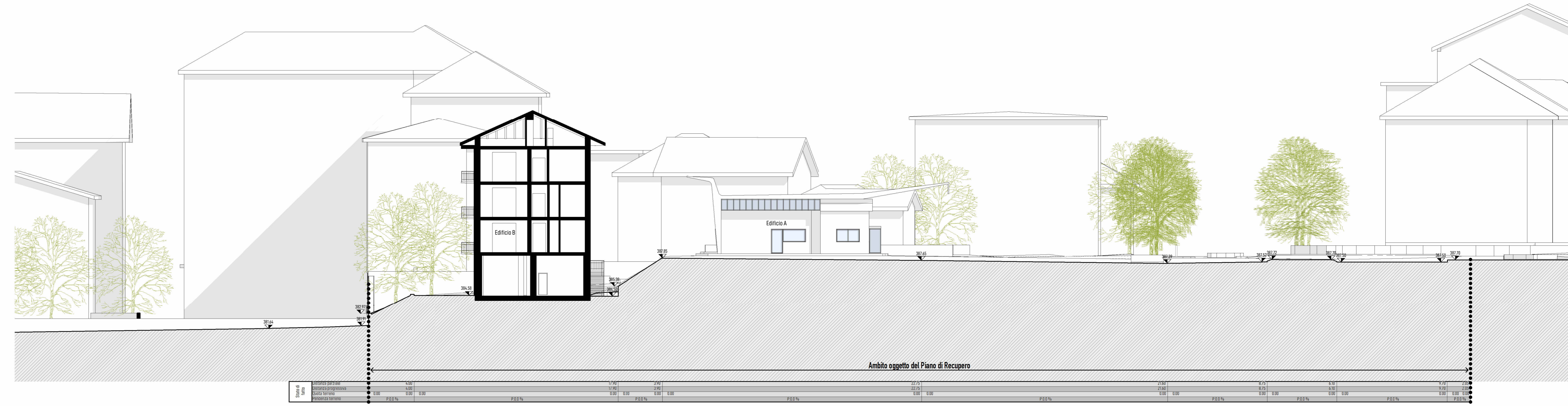
Sezione GG - 1:200
