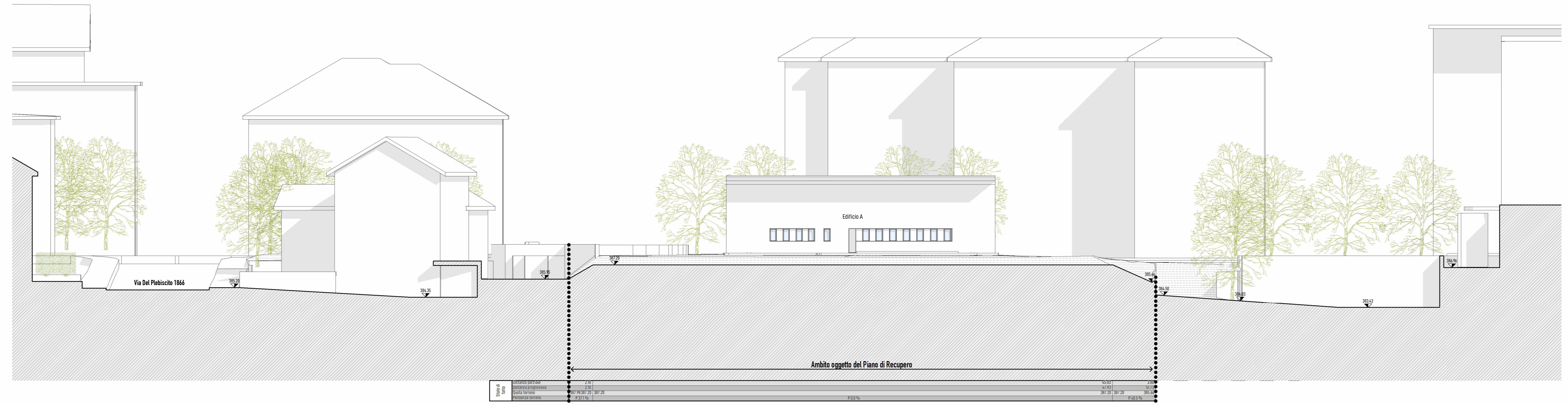
Sezione CC - 1:200
