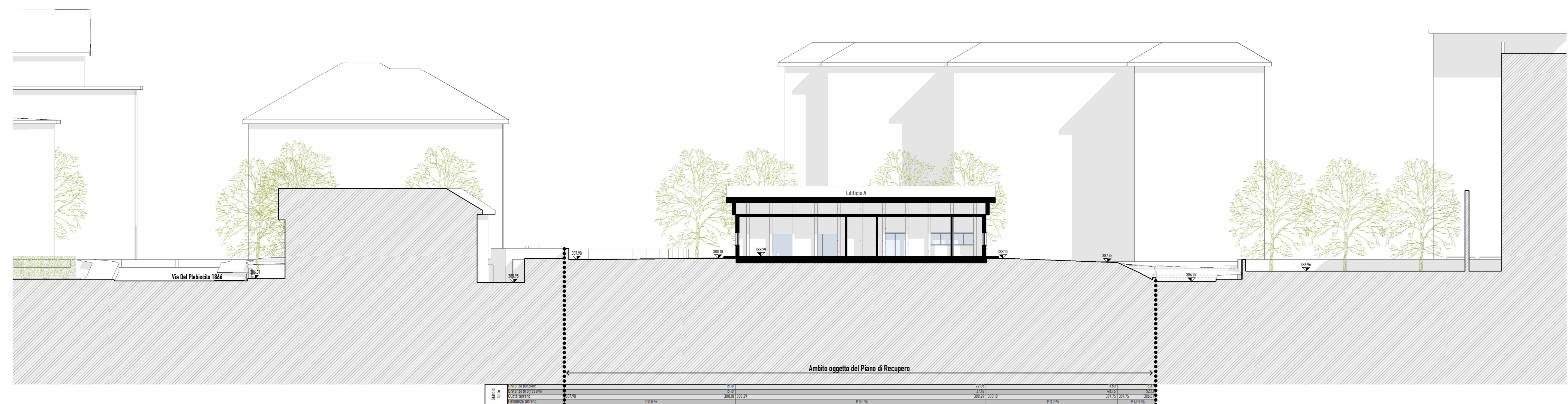
Sezione BB - 1:200
