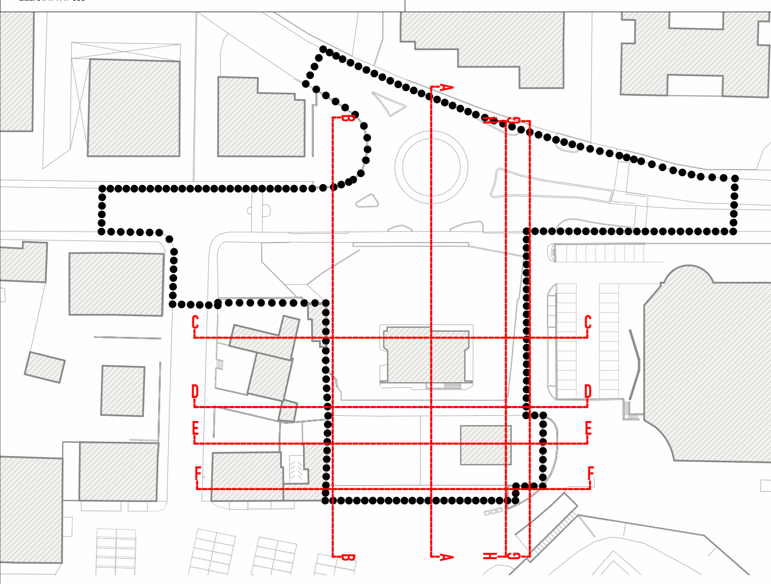
Inquadramento - 1:1000
