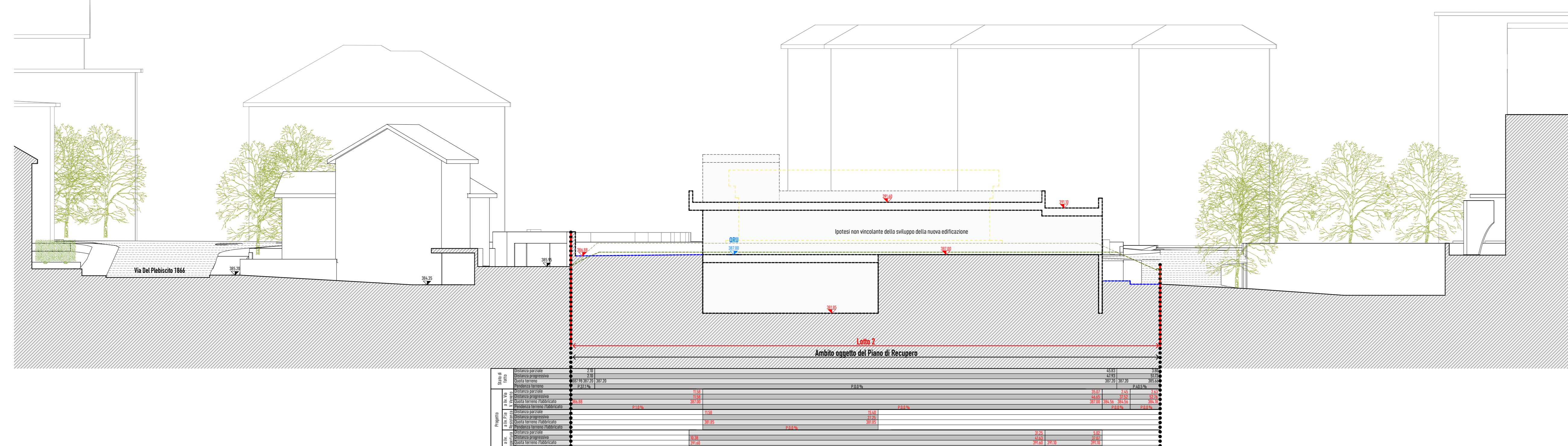
Sezione DD - 1:200
