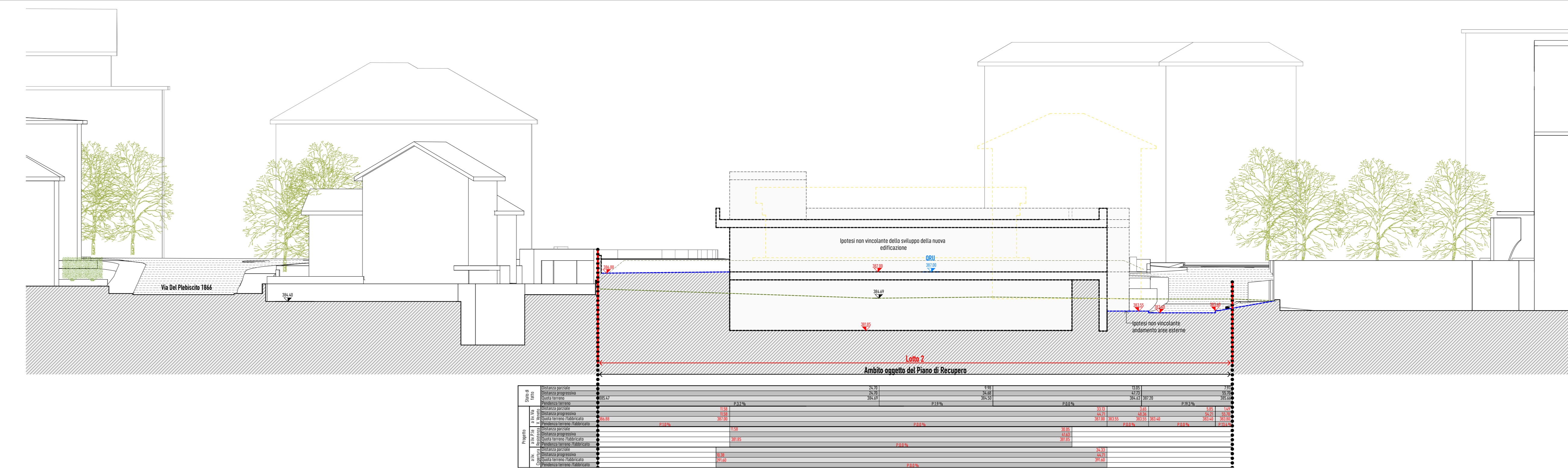
Sezione EE - 1:200
