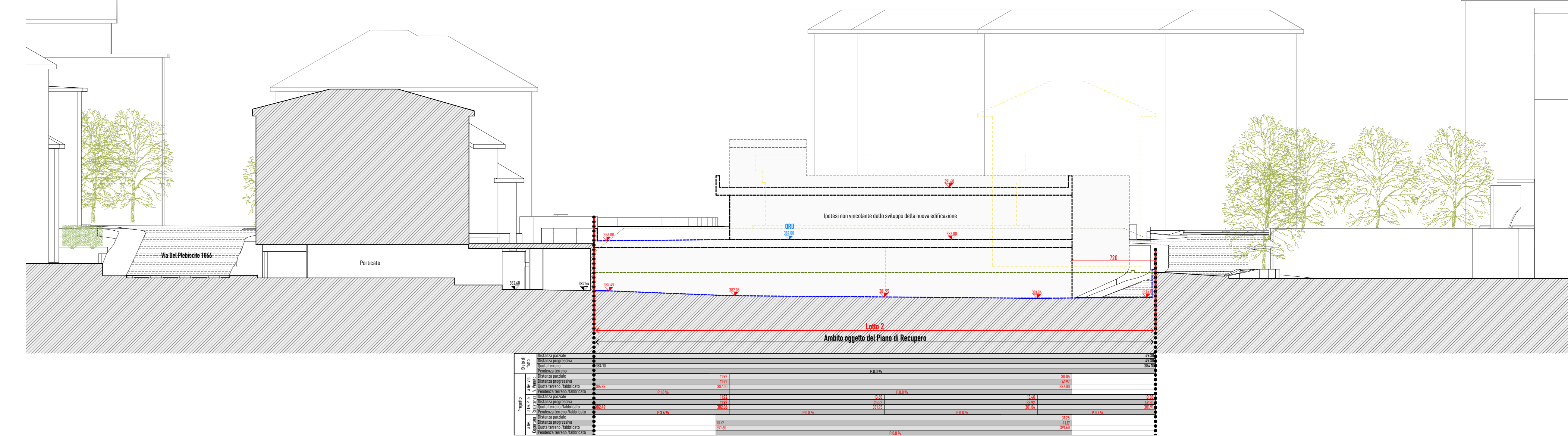
Sezione FF - 1:200
