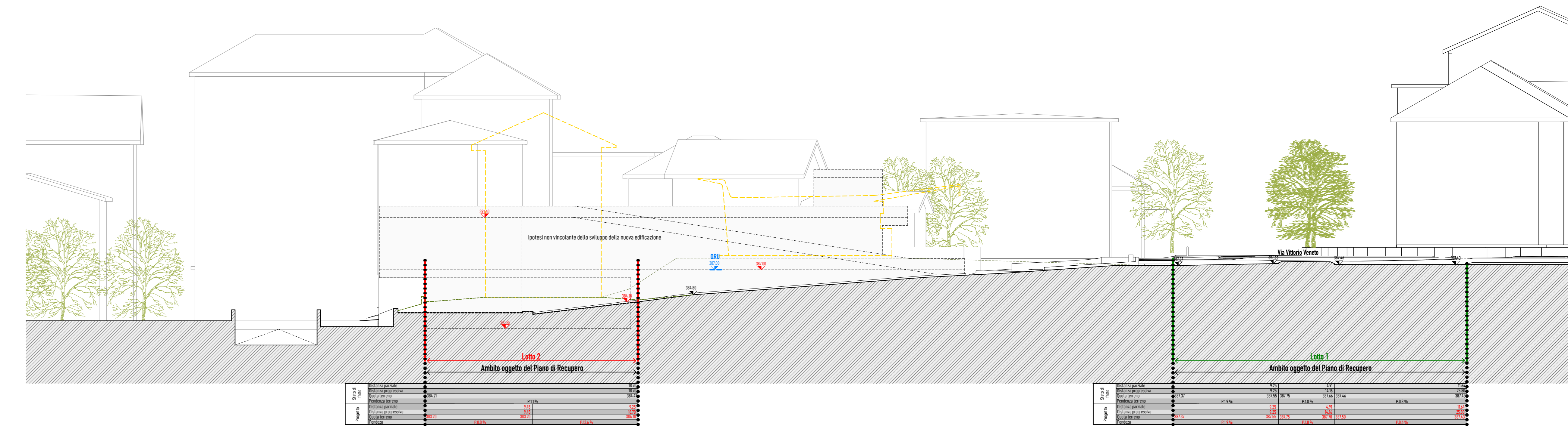
Sezione GG - 1:200
