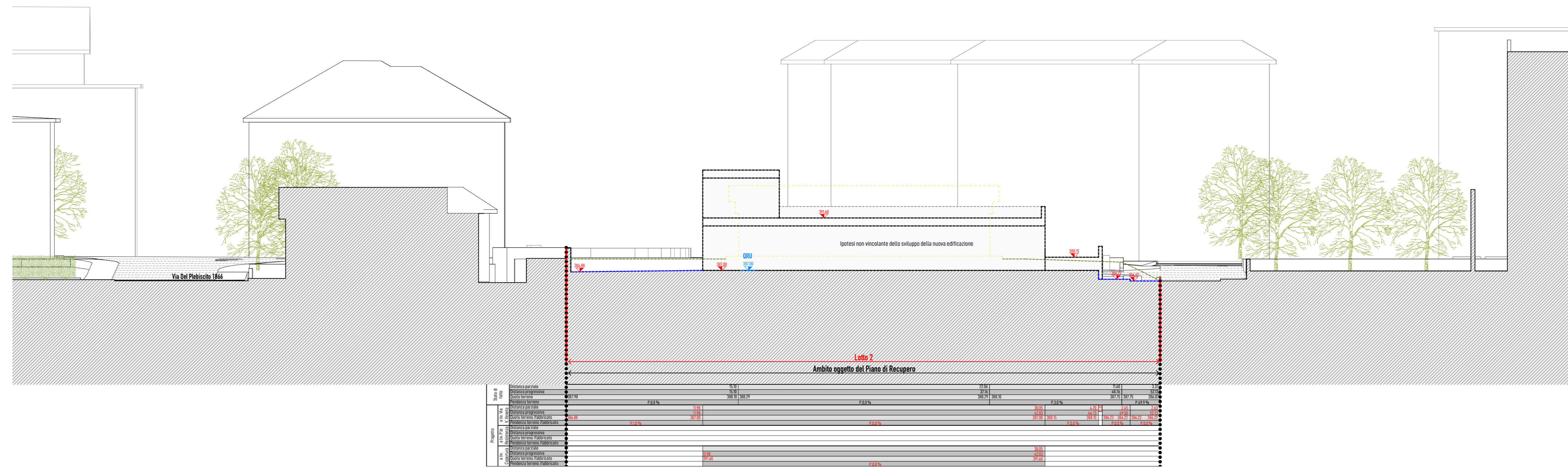
Sezione CC - 1:200
