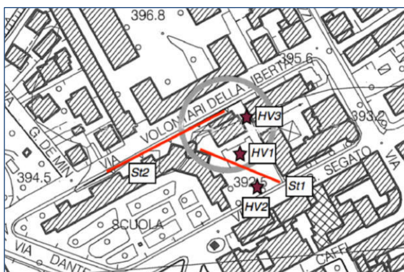
Figura 36 - ubicazione indagine geofisica Via Segato (FONTE: comune di Belluno, RELAZIONE Geologica Via Segato Scuola Gabelli, 2015- vedi BIBLIOGRAFIA)
