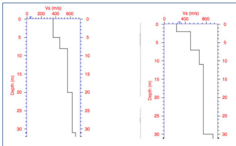
Figura 28 - profili sismici FTAN S1 e S2 (FONTE: comune di Belluno, Caratterizzazione sismica scuola elementare Levego, Dr. Boaga, 2011 - vedi BIBLIOGRAFIA)
