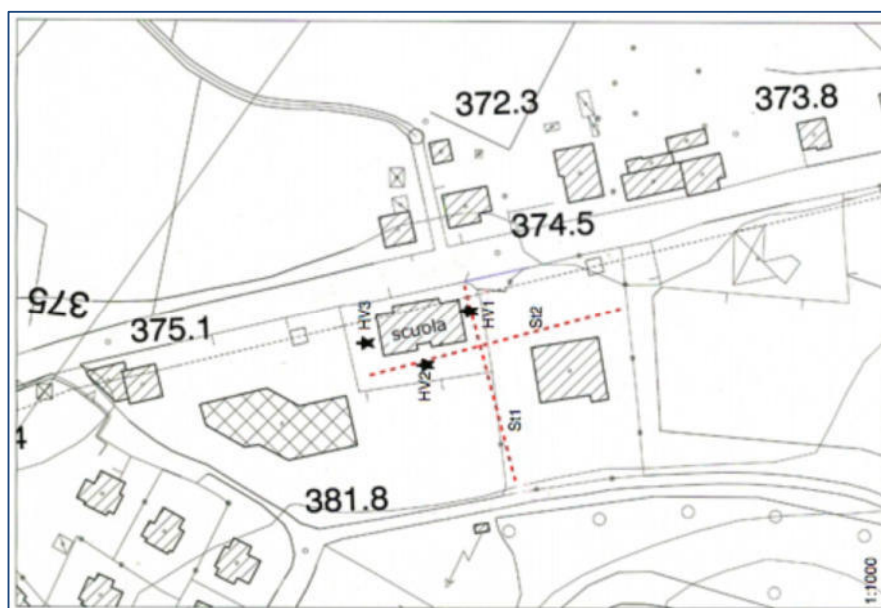
Figura 27 - ubicazione indagini geofisiche Fraz. Levego
