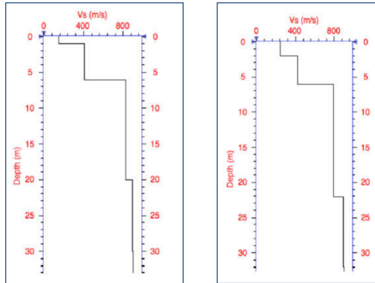
Figura 37 - profilo sismico S1 (FONTE: comune di Belluno, RELAZIONE Geologica Via Segato Scuola Gabelli, 2015- vedi BIBLIOGRAFIA)
