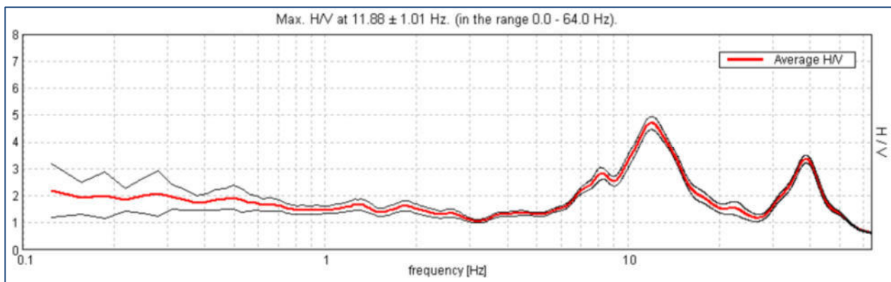
Figura 35 - profilo sismico HVSR1 (FONTE: comune di Belluno, indagine geologica Frazione Levego Via Meassa - vedi BIBLIOGRAFIA)
