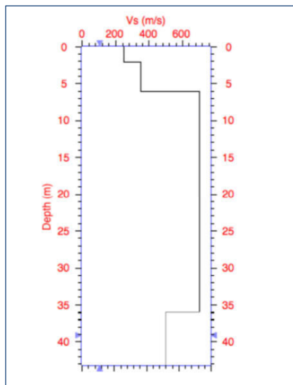
Figura 34 - profilo sismico S1 (FONTE: comune di Belluno, indagine geologica Frazione Levego Via Meassa - vedi BIBLIOGRAFIA)
