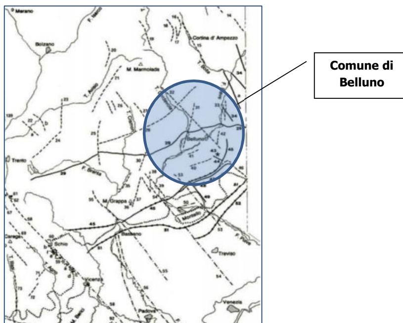
Figura 15 - Carta generale delle faglie attive del sud-alpino centro orientale (FONTE: Castaldini-Panizza 1991)
