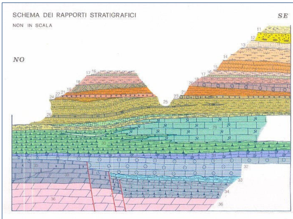
Figura 24 - Schema dei rapporti stratigrafici delle formazioni mesozoiche affioranti nel bellunese tramite una sezione ideale. Le superfici oblique sulla destra dello schema rappresentano la scarpata della Piattaforma Friulana (FONTE: Carta Geologica F. 063 "Belluno" del Progetto CARG)
