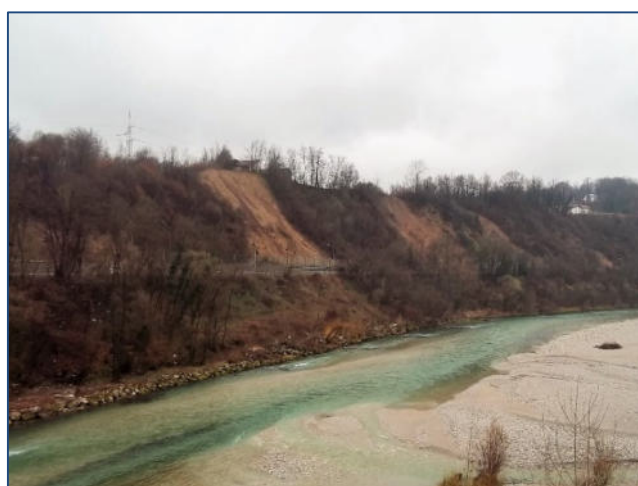
Figura 23 – frane sul terrazzo (orli di scarpata) in sinistra orografica del Piave nell'area a valle del Col Cavalier, foto di Antonio Toscano
