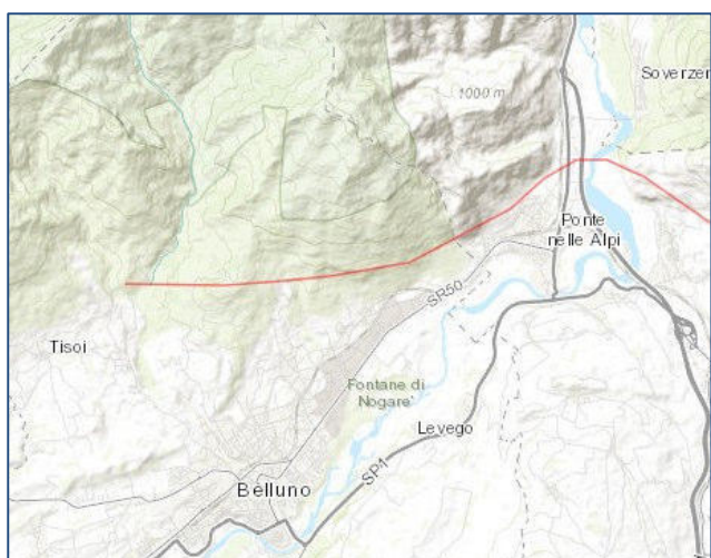
Figura 53 - Traccia della linea di faglia (FONTE: PROGETTO ITHACA)
