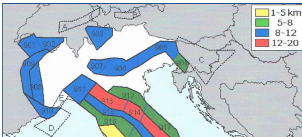
Figura 6 - Classi di profondità efficace assegnate alle diverse zone ZS sulla base dei valori della moda e della forma della frequenza degli eventi in funzione della profondità (FONTE: GRUPPO DI LAVORO I.N.G.V.)
