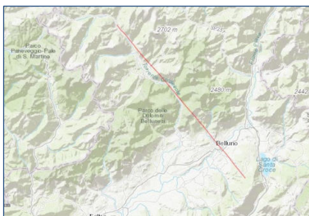
Figura 51 - Traccia della linea di faglia (FONTE: PROGETTO ITHACA)
