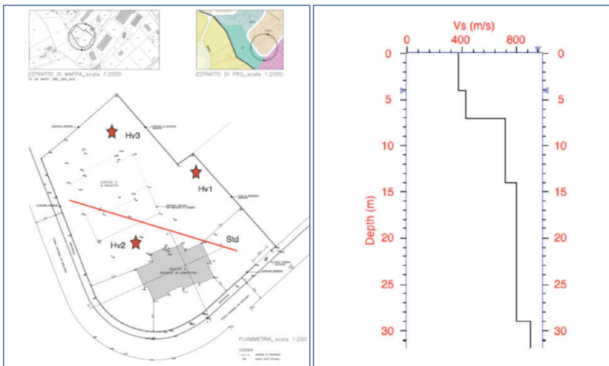
Figura 30 - ubicazione profilo sismico
