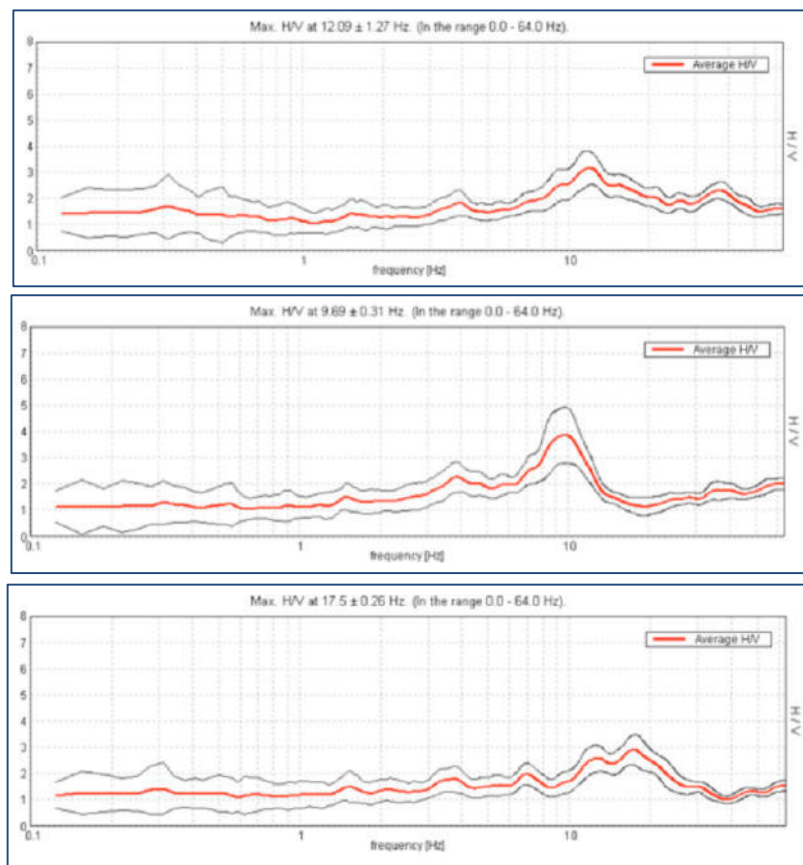
Figura 38 - profili sismici HVSR1 HVSR2 HVSR3 (FONTE: comune di Belluno, RELAZIONE Geologica Via Segato Scuola Gabelli, 2015 - vedi BIBLIOGRAFIA)
