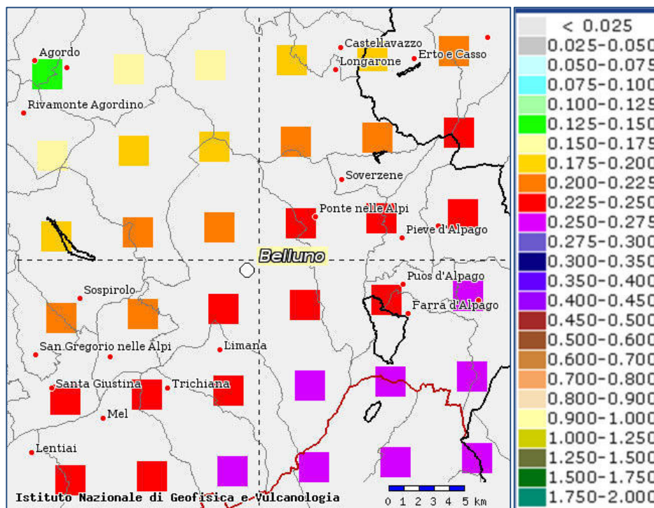
Figura 71 - Mappa interattiva di pericolosità sismica redatta a cura dell'INGV di Milano Punti della griglia riferiti a: parametro dello scuotimento a_g ; probabilità in 50 anni 10%; percentile 50 (FONTE http://esse1-gis.mi.ingv.it/ )
