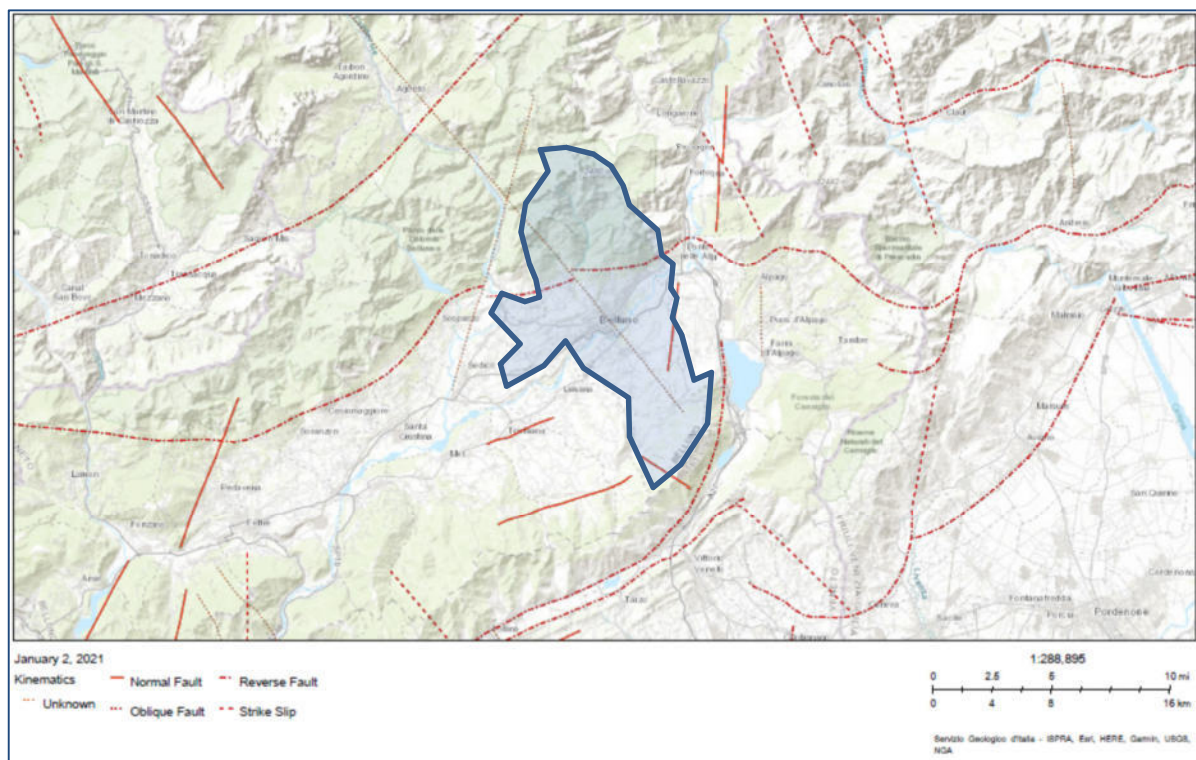
Figura 16 - Stralcio della Carta delle FAGLIE CAPACI 22 BELLUNO IN BLU (FONTE: ITHACA "ITaly Hazard from CAPable faults")
