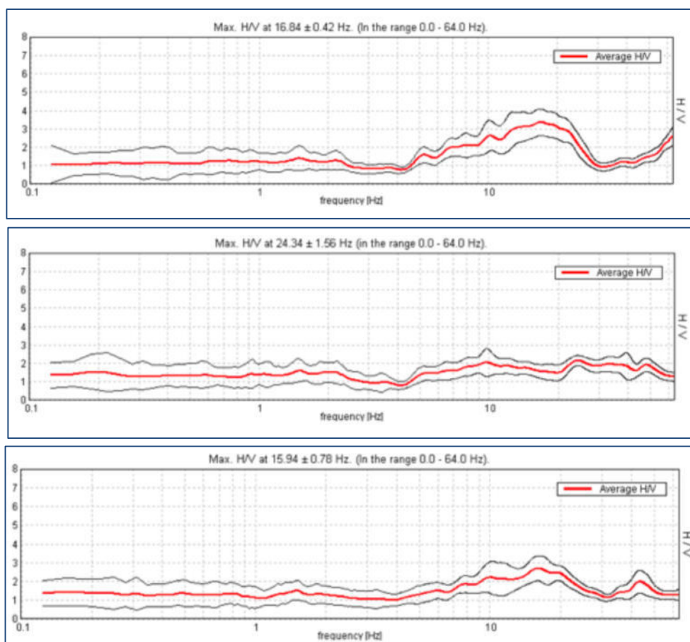
Figura 29 - profili sismici HVS1 - HVS2 - HVS3 (FONTE: comune di Belluno, Caratterizzazione sismica scuola elementare Levego, Dr. Boaga, 2011 - vedi BIBLIOGRAFIA)
