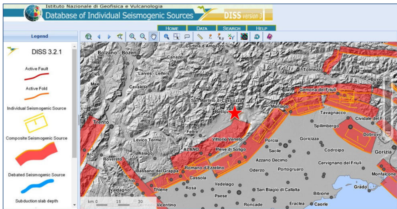
Figura 7 - Database of Individual Seismogenic Sources dell'INGV (FONTE: DISS http://diss.rm.ingv.it/dissmap/dissmap.phtml ) ubicazione comune di Belluno:
