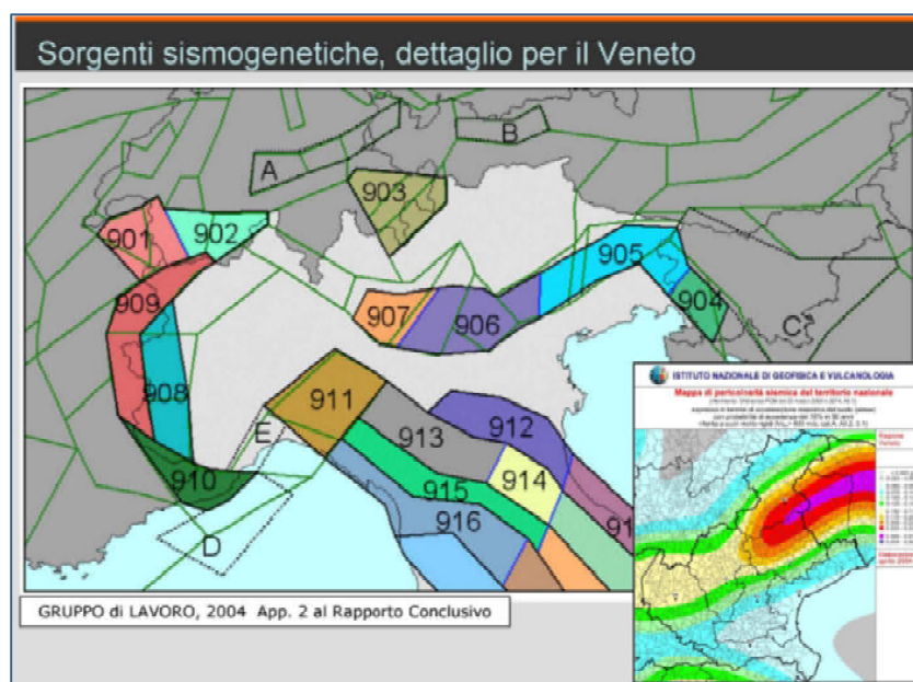
Figura 4 - Particolare della zonazione sismogenetica - Italia settentrionale (FONTE: INGV- AA.VV. 2004)
