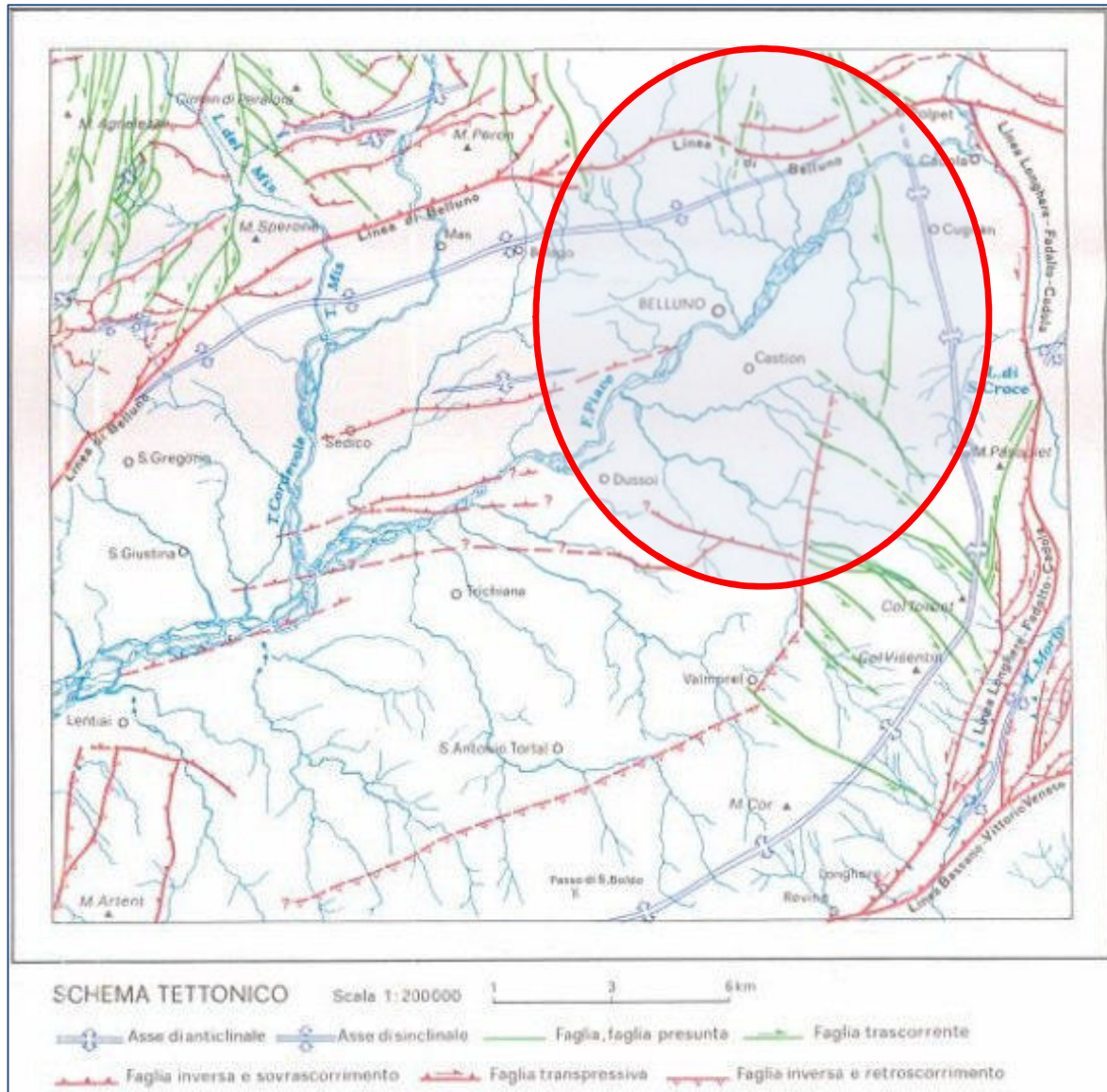
Figura 25 - schema tettonico area in esame (FONTE: foglio geologico CARG N.63 "Belluno")
