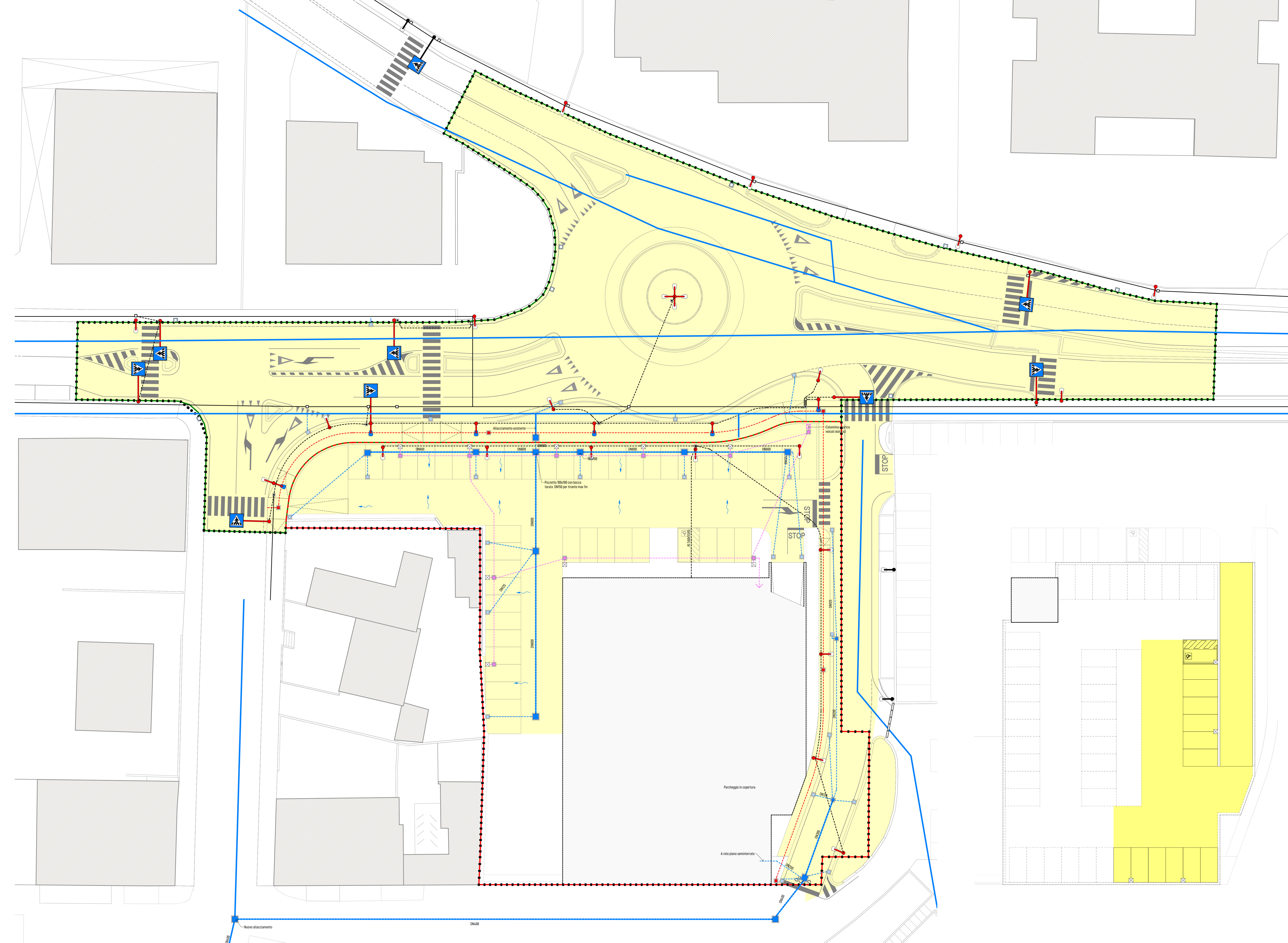
Planimetria generale d'ambito con indicate le previsioni di piano a livello di via Vittorio Veneto
