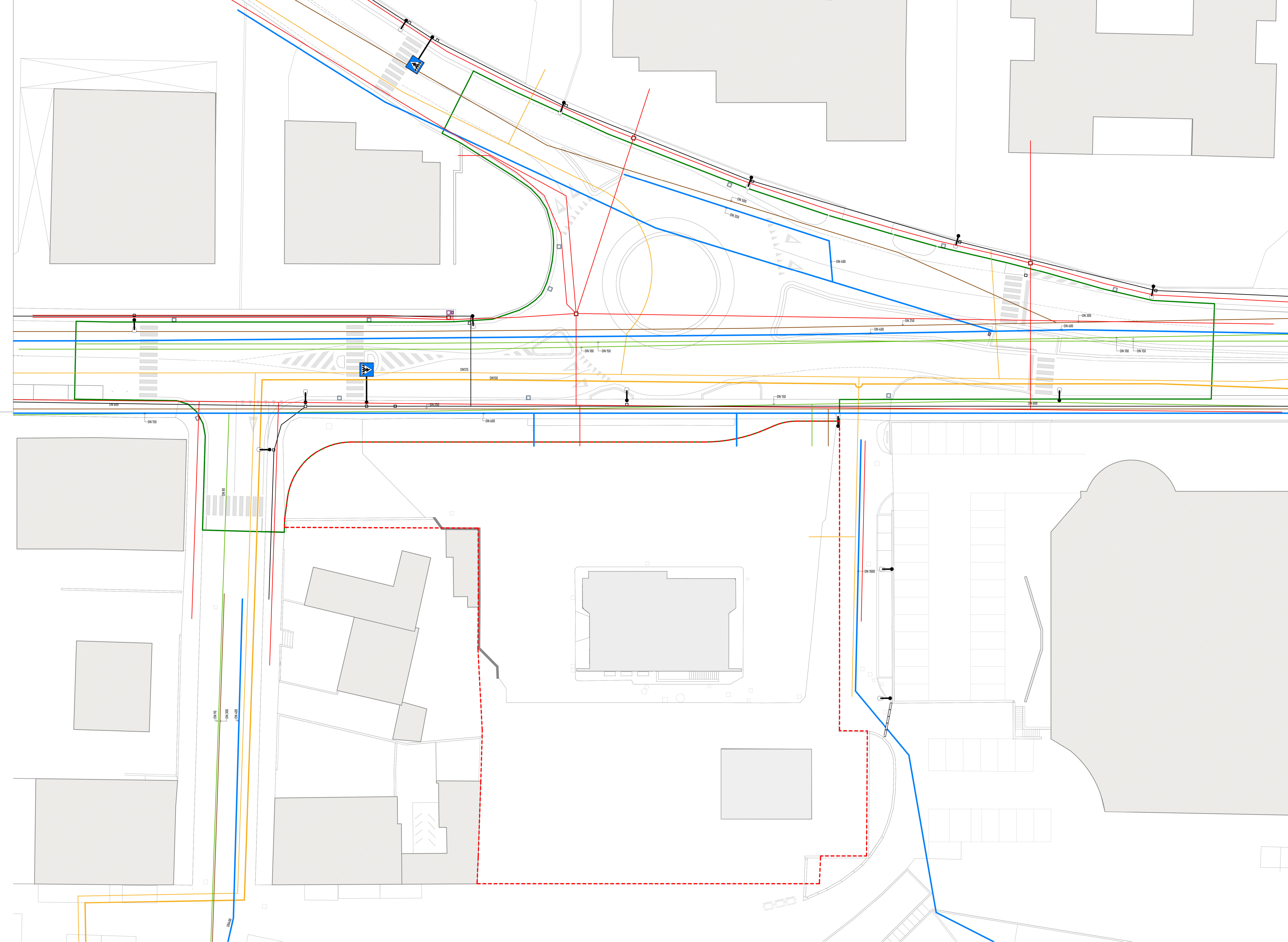
Planimetria stato di fatto con indicate le reti esistenti
