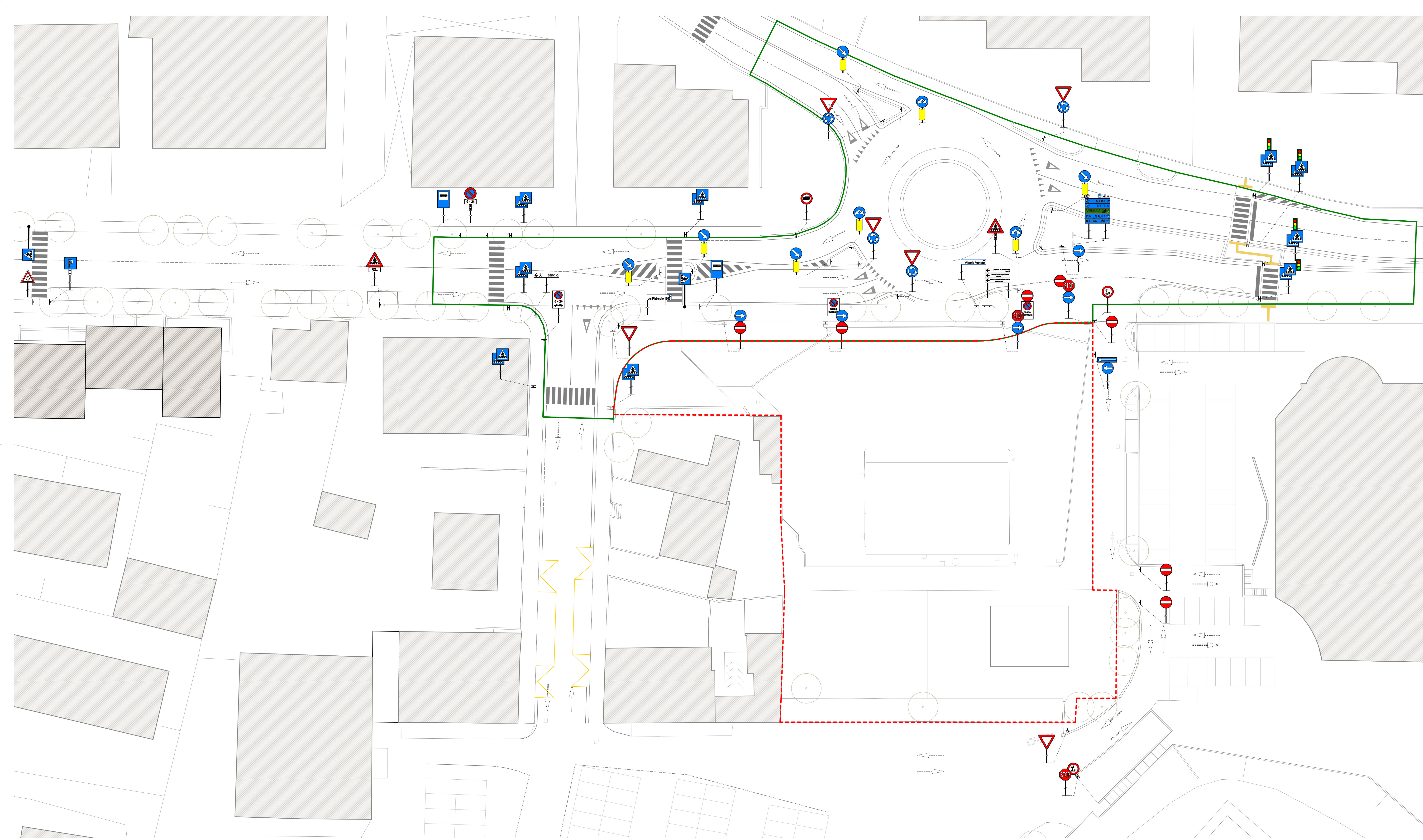
Planimetria generale stato di fatto
