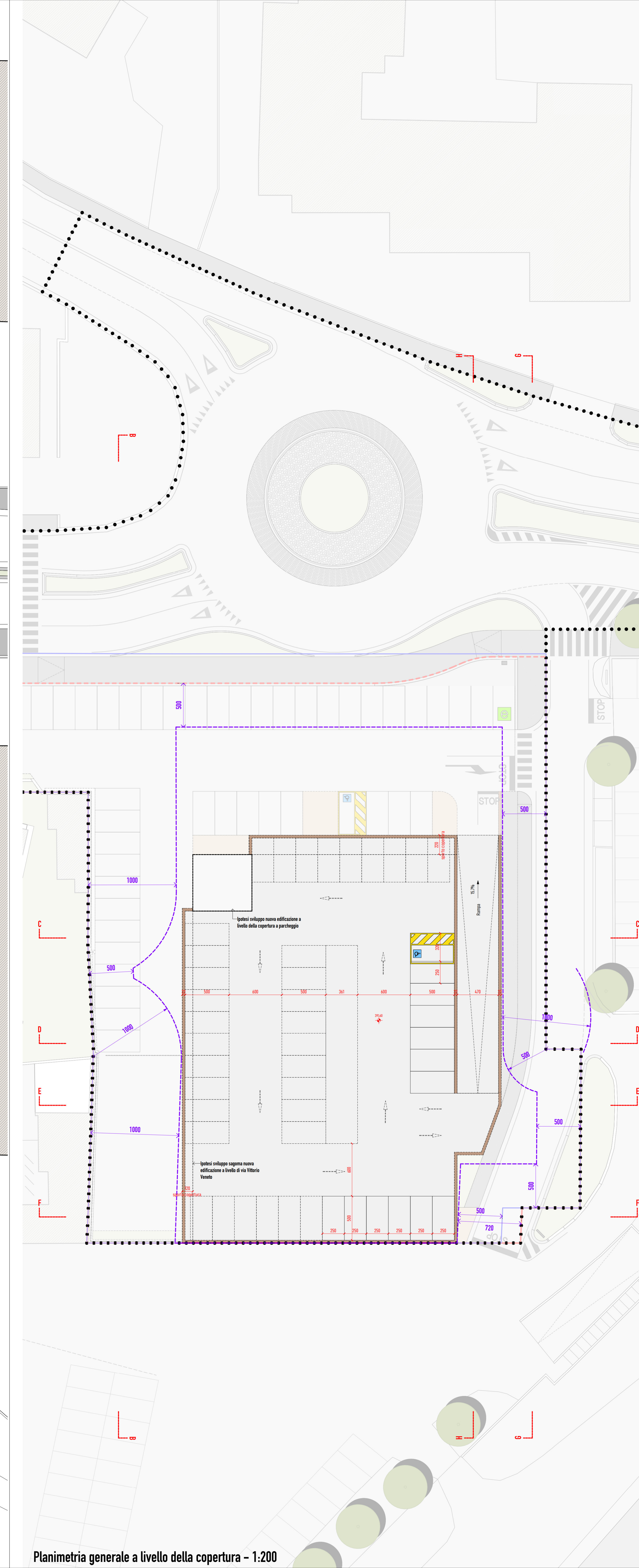
Planimetria generale a livello della copertura - 1:200
