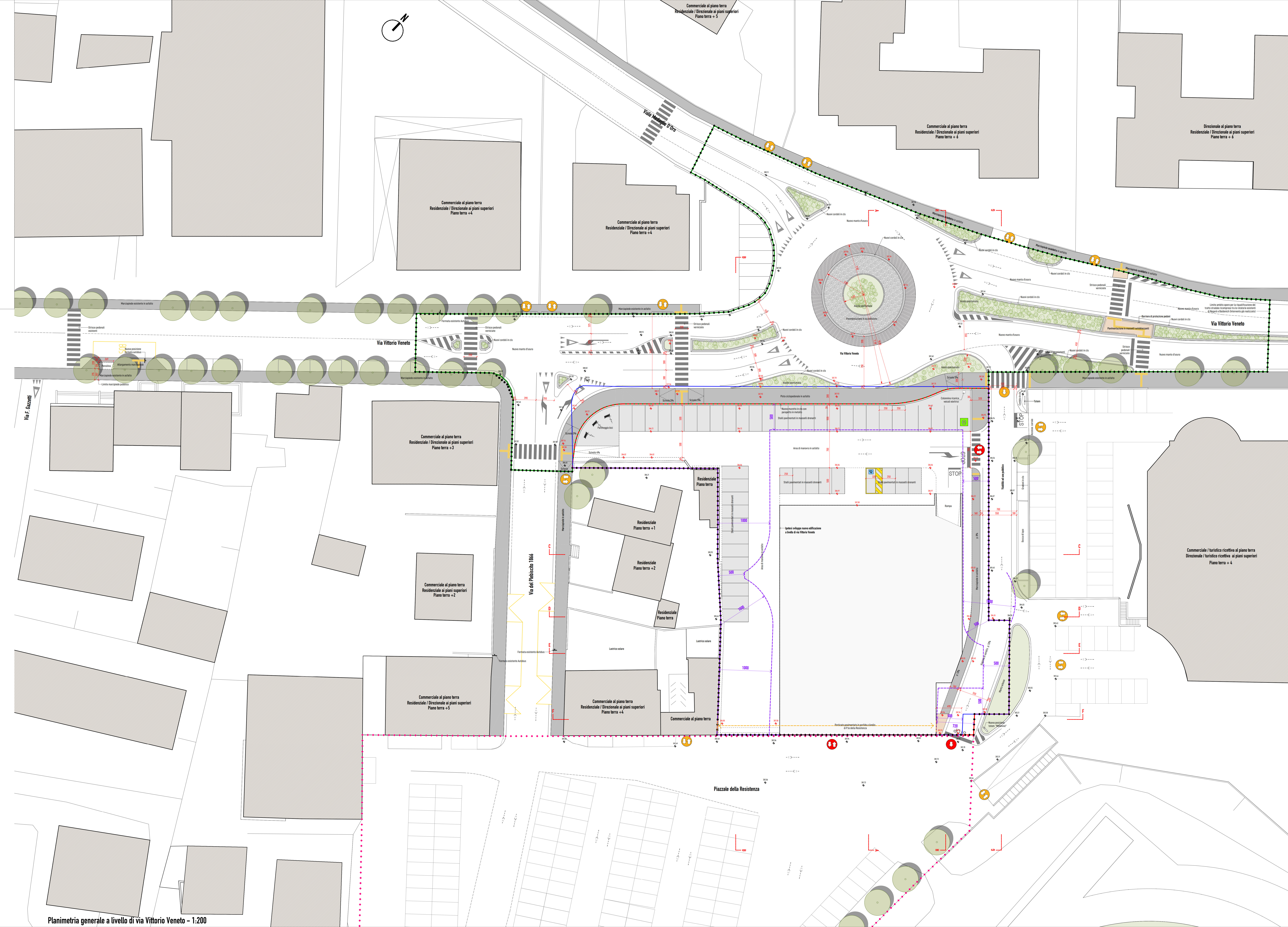
Planimetria generale a livello di via Vittorio Veneto - 1:200
