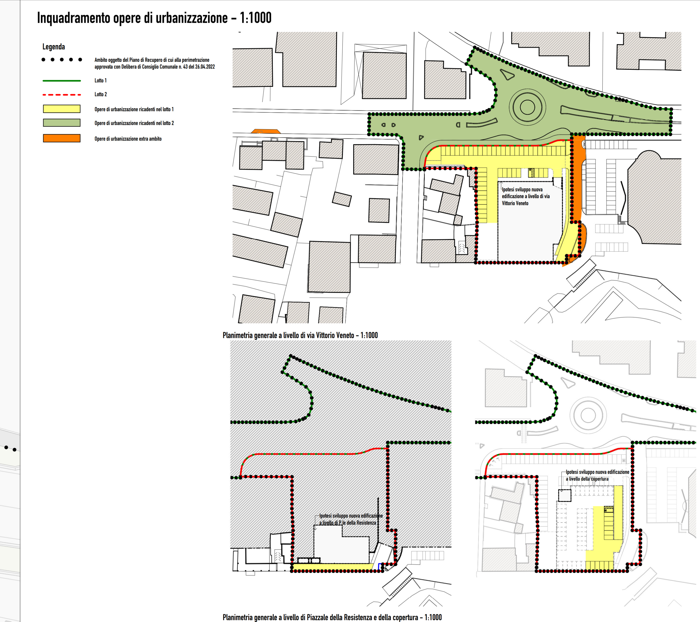
Planimetria generale a livello di Piazzale della Resistenza e della copertura - 1:1000
